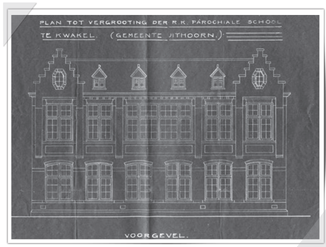
Bouwtekening Stegerhoek (1919)
